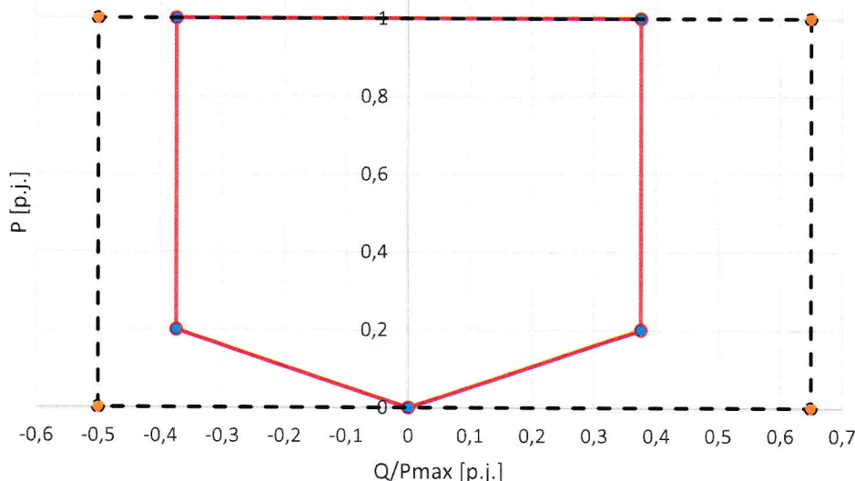
Obr. 3 Diagram dodávky jalového výkonu při nižší než maximální dodávce činného výkonu pro nesynchronní výrobní moduly kategorie D
