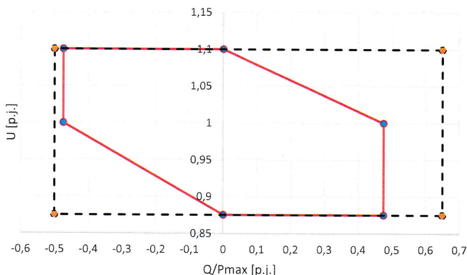
Obr. 1 Diagram dodávky jalového výkonu při maximální dodávce činného výkonu pro synchronní výrobní moduly kategorie D
