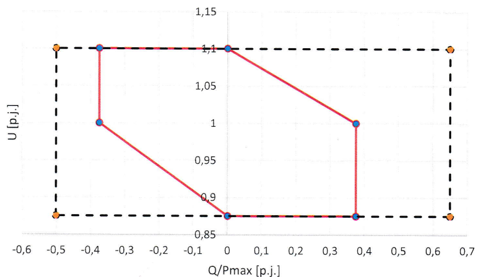
Obr. 2 Diagram dodávky jalového výkonu při maximální dodávce činného výkonu pro nesynchronní výrobní moduly kategorie D
